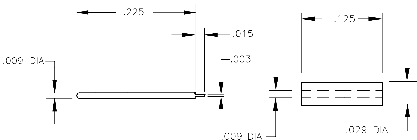
PIN/TAB 1490-02P
