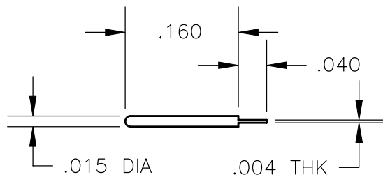
PIN/TAB 290-25P
