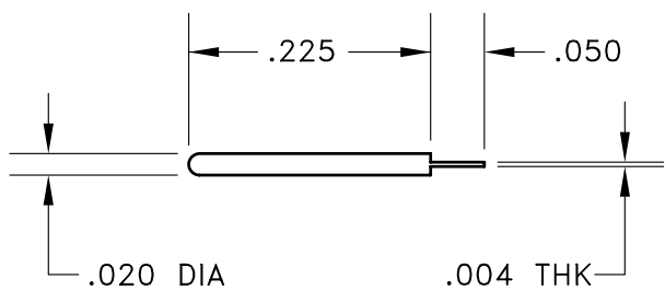
PIN/TAB 290-26P
